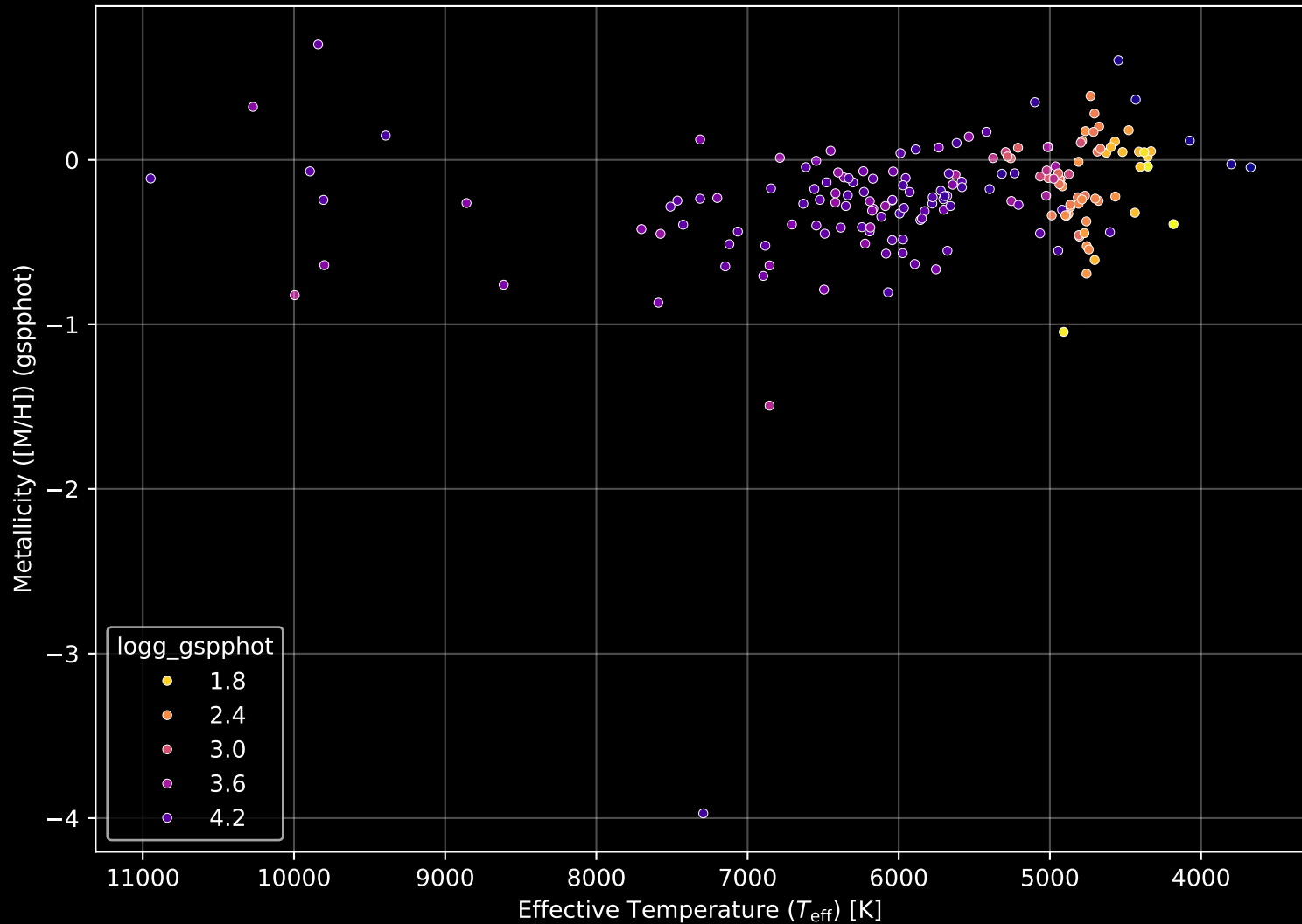
APOGEE DR17 Field: [CVZ_OB03_btx] Stellar Population Parameters (n= 179)
